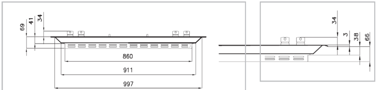
FT Disegno tecnico della versione Filotop Technical drawing of Flush-mount version
